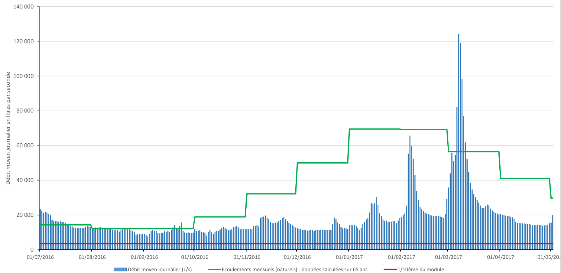
Représentation du type d'observation Débit moyen journalier à la station hydrométrique M050062001 - La Sarthe à Spay [aval]
