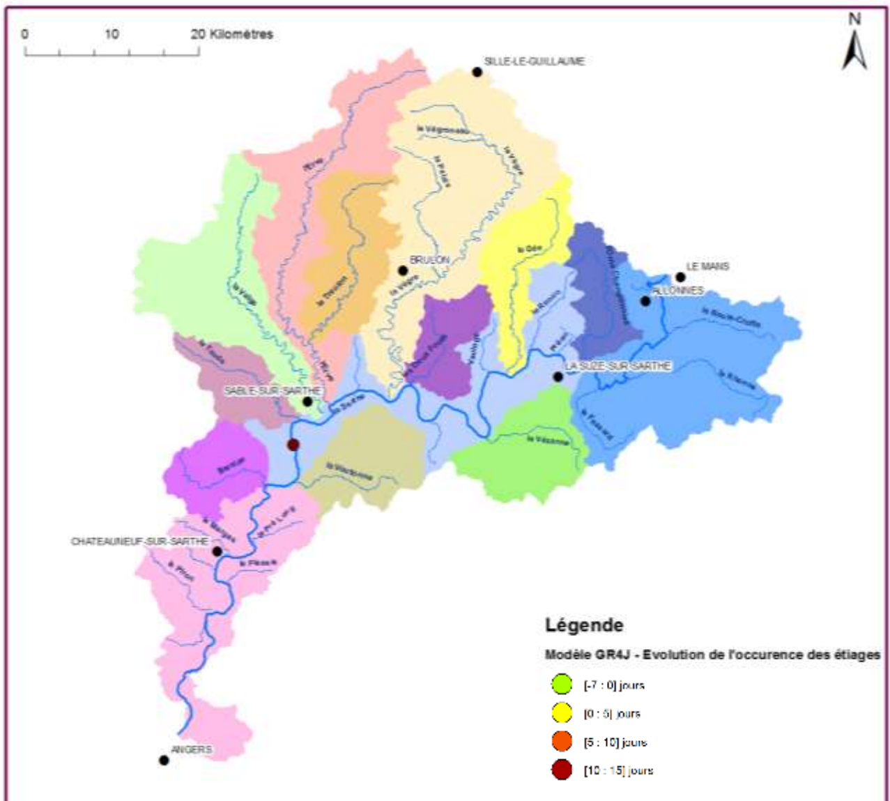
Figure 8-3 : Évolution des occurrences des sécheresses à horizon 2045-2065 pour le modèle GR4J
