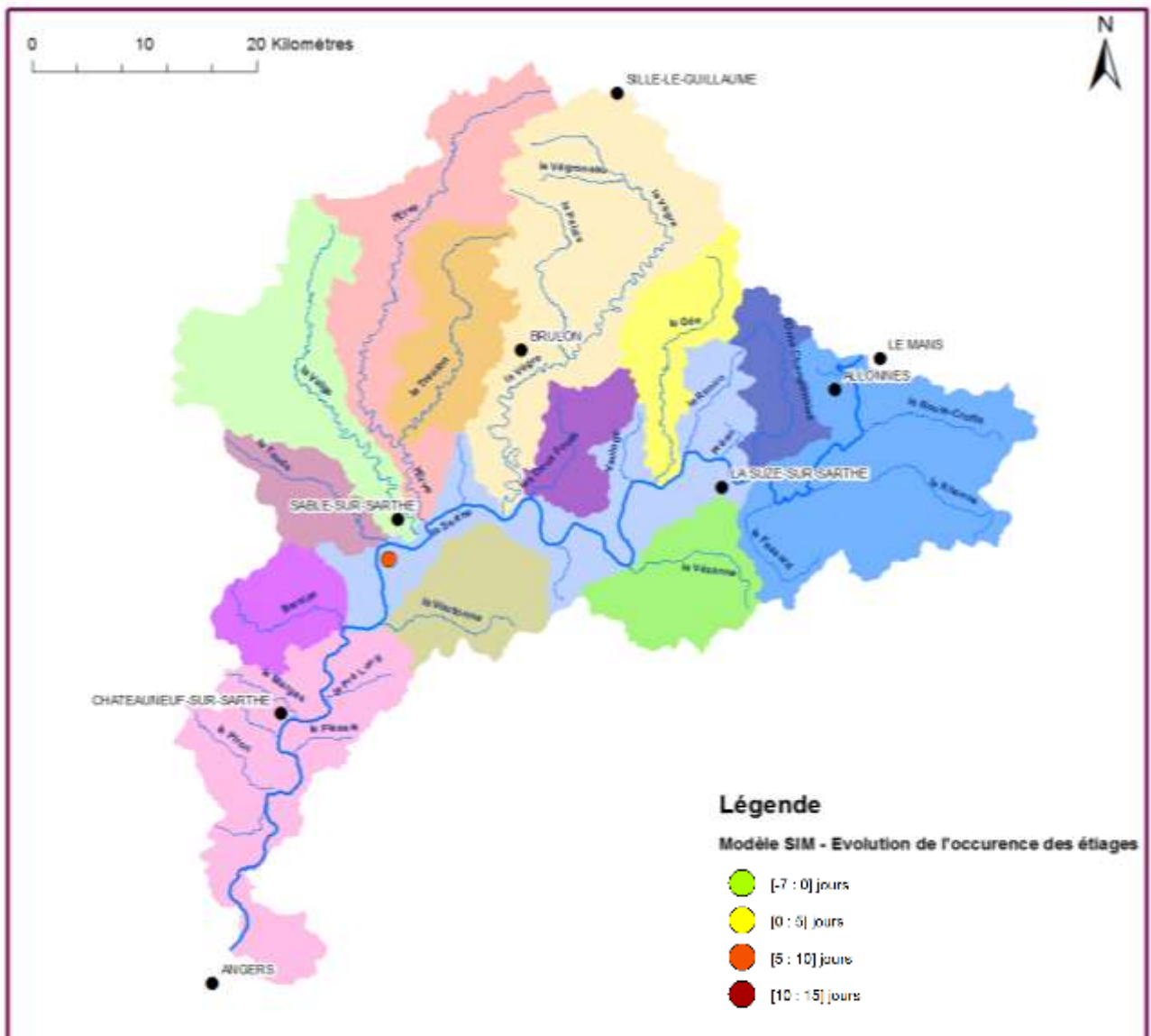
Figure 8-4 : Évolution des occurrences des sécheresses à horizon 20456-2065 pour le modèle SIM
