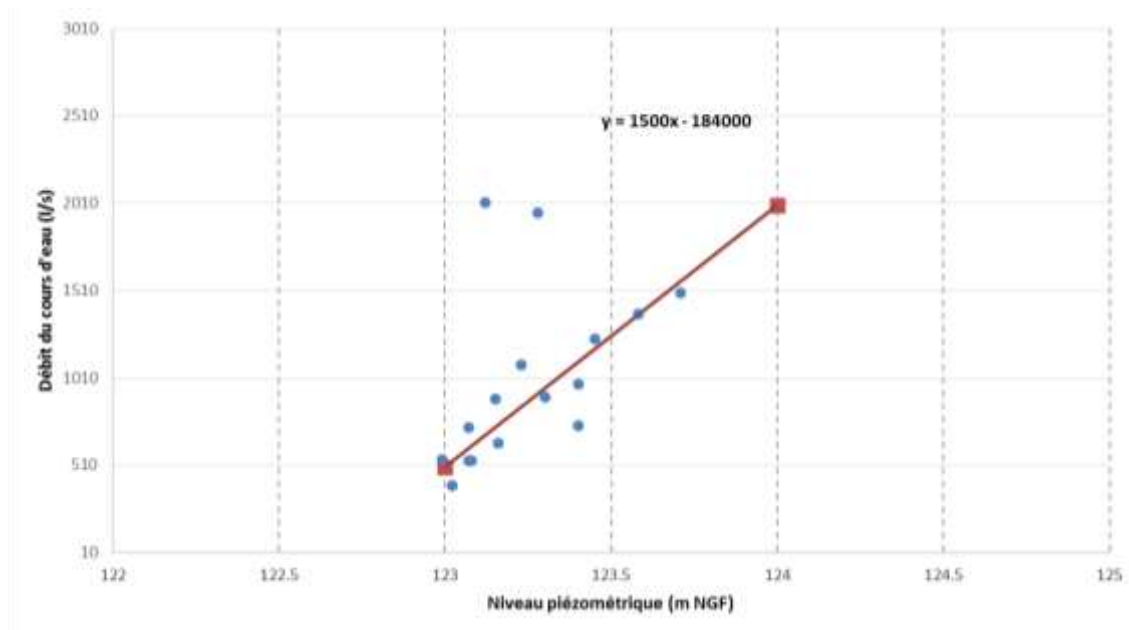
Figure 7-2 : Comparaison des types de corrélation (A, B et C) Niveau piézométrique – Débit rivière
