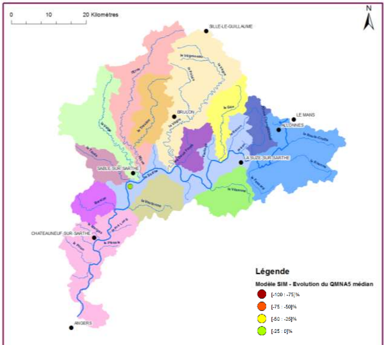
Figure 8-2 : Évolution du QMNA5 médian à horizon 20456-2065 pour le modèle SIM
