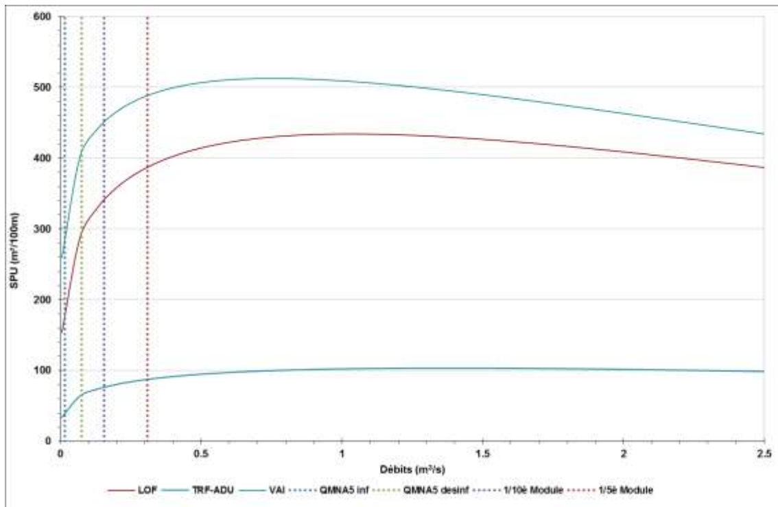
Figure 2-11 : Évolution de la Surface Pondérée Utile sur le secteur de la Vaige (LOF = Loche Franche / TRF-ADU = Truite fario adulte / VAI = Vairon)
