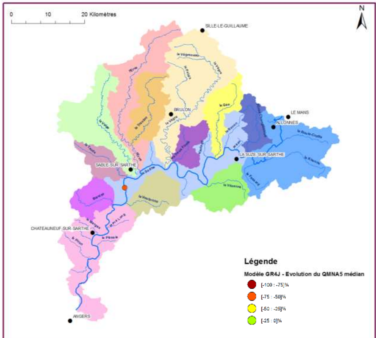
Figure 8-1 : Évolution du QMNA5 médian à horizon 20456-2065 pour le modèle GR4J
