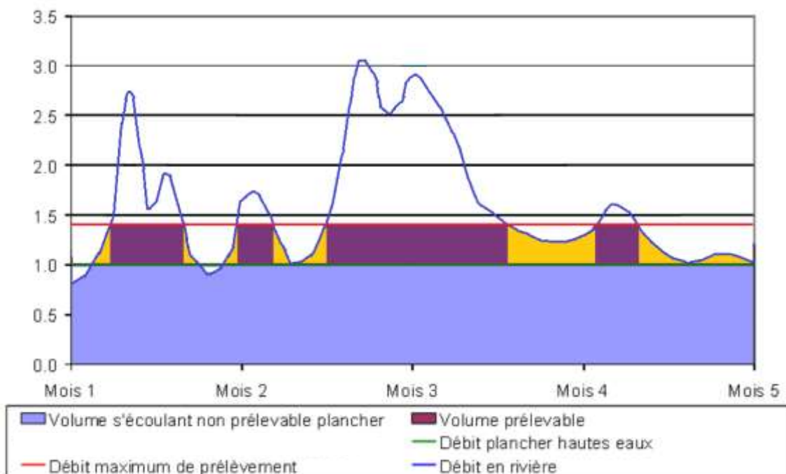
Figure 3-1 : Schéma de principe pour le calcul du volume prélevable en période de hautes eaux
