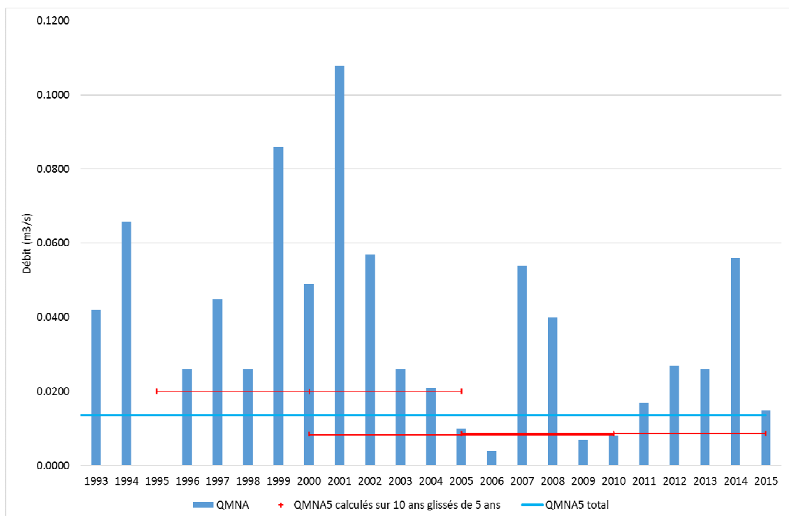
Figure 3-10 : Stationnarité des débits caractéristiques d'étiage à la station hydrométriques sur la Vézanne à Malicorne-sur-Sarthe
