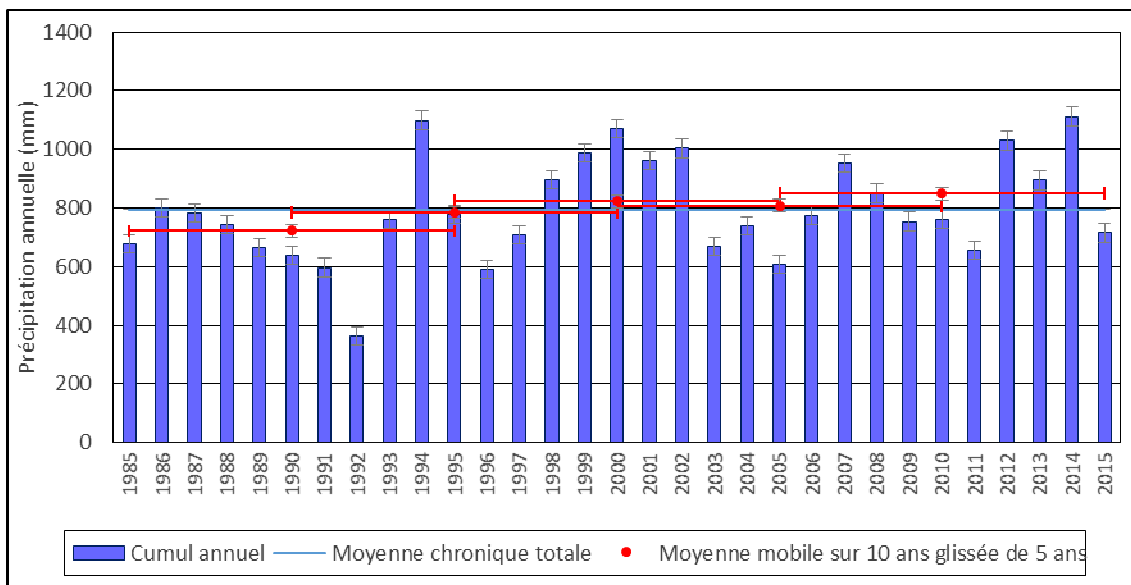
Figure 2-13 : Comparaison des cumuls de pluie annuels et des moyennes mobiles sur 10 ans sur toute la période disponible à la station de Tennie
